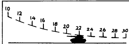
ציור מס' 3: משפך טווחים. בציור נראה טנק ש"נתפס" בטווח 2200 מ'. המספר 2.7 מתחת לקו מציינן שהמשפך מתאים למטרות שגובהן 2.7 מ'.
