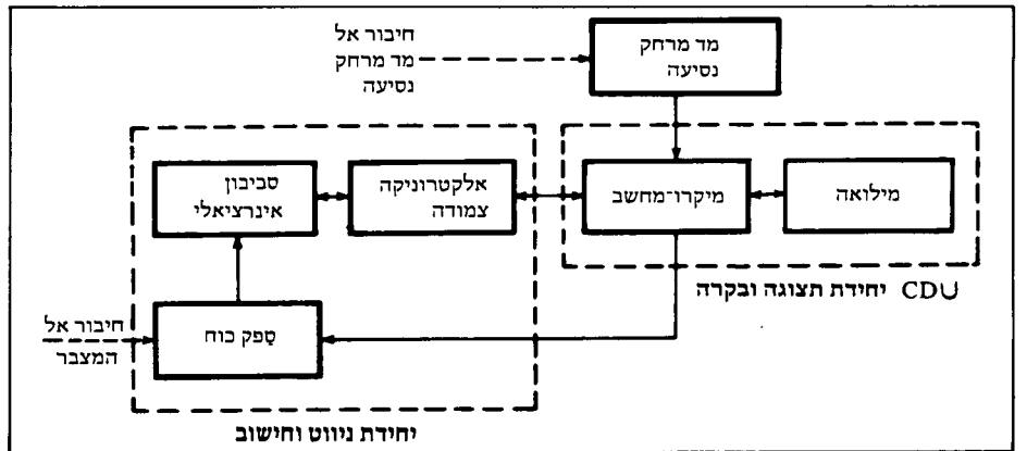
מערכת "לאנס" — תיאור כללי
