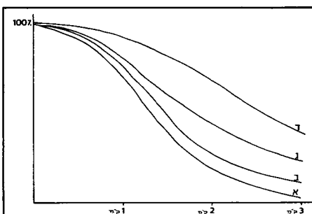
צויר מס' 6: סכימה של סיכויי הפגיעה בכדור ראשון, בתחמושת נ"ט כלפי מטרת טנק, בתלות טווח: א. בטנק סנטוריון ללא מד-טווח; ב. בטנק פאטון עם מד טווח אופטי; ג. בטנק M60A3 עם מחשב ירי, מד טווח לייזר ועוד; ד. בטנק XM-1 מבין המשוכללים ביותר כיום.
