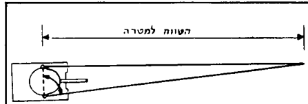
ציור מס' 2: פעולתו של מדיטווח אופטי מבוססת על התלכדות קווי הראייה אל המטרה. קווי-הראייה יוצאים מקצוות מד הטווח בשני צדי הצריח. עפ"י הזווית המשתנה (מסומנת בקשת) נקבע הטווח למטרה.
