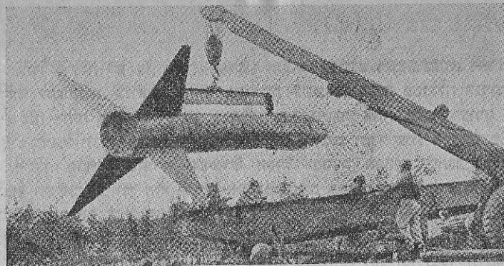
ההטענה
