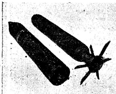
קלעירקטות שבשימוש צבא ארה"ב מימין: קלעירקטה M 8; קוטרו 4.5 אינץ משמאל: קלעירקטה M 16; קוטרו 4.5 אינץ
