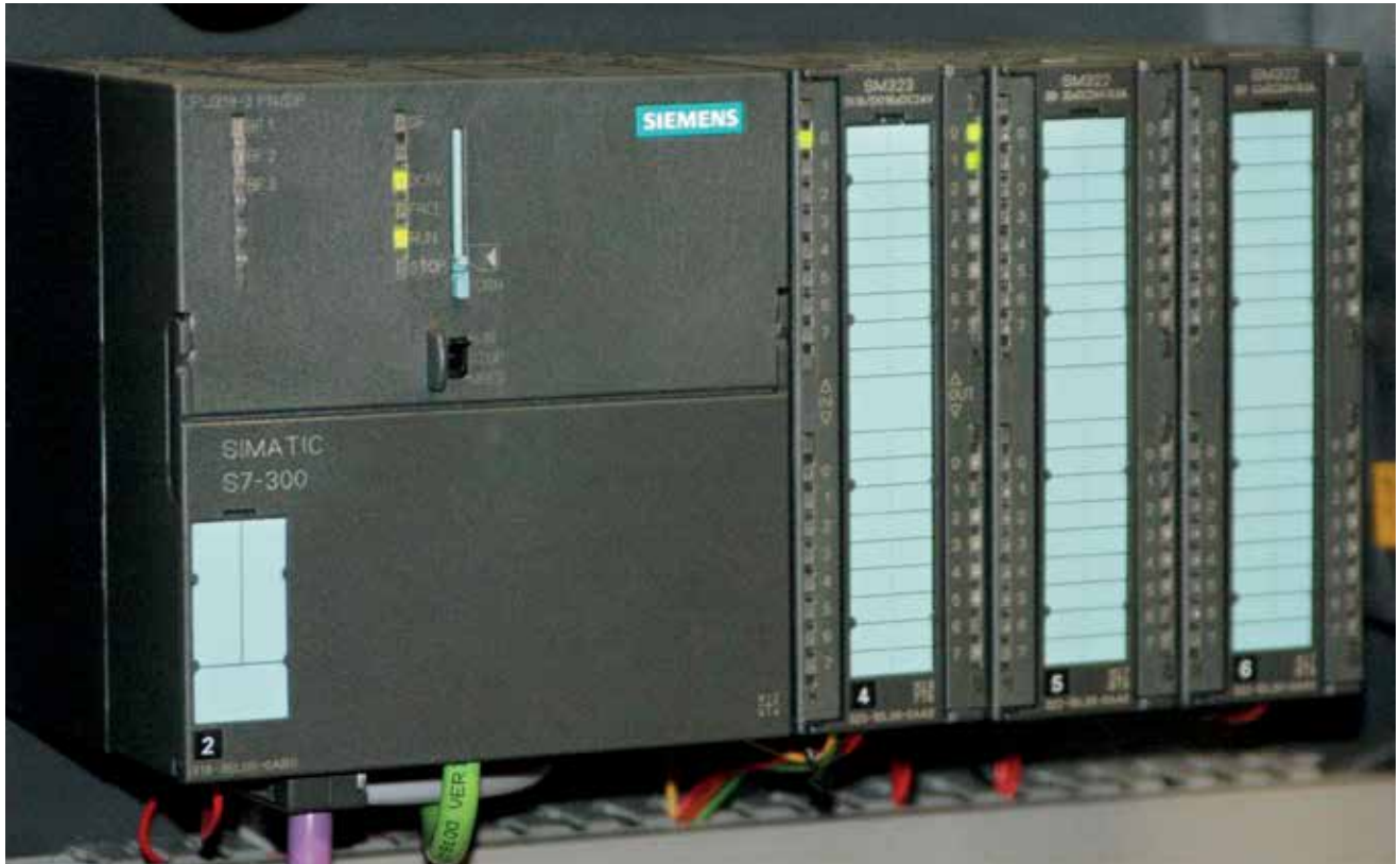
מערכת הבקרה של הצנטריפוגות שעמדה במוקד המחקפה של סטוקסנט. גורם זר הצליח ככל הנראה להחדיר נוזקה מסוג סטוקסנט לתוך מחשבו האישי של מהנדס איראני שעבד בתוכנית הגרעין האיראנית
