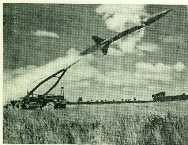
„יוחנן הישר“ מזנק מכן השיגור הנייד, בנושא ראש נפץ אווירי. יש בכוחו של הטיל, שאורכו 8.2 מ', להרוס עיר קטנה הנמצאת במרחק של כ-26 ק"מ.
