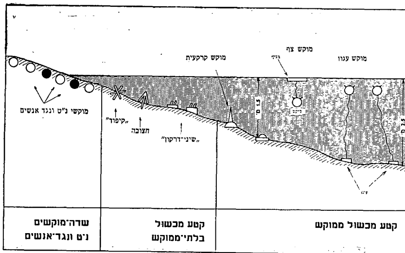
מרשם מס' 4: תכנית מכשול
