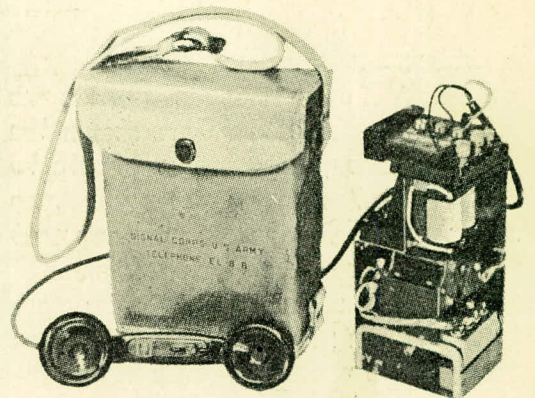
טלפון-שדה בצבא ארה"ב, נתון במעטה ברונזי; משקלו 9,5 ליברות.
