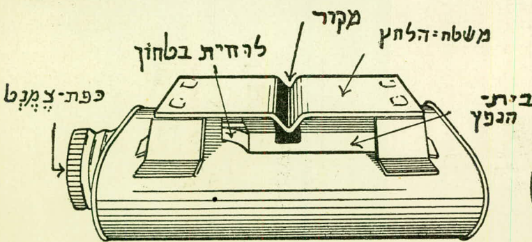
רימון-המוקש הבריטי מס' 75
