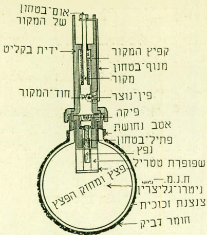
רימון דביק אנטי-טנקי מס' 71 (בריטי)
