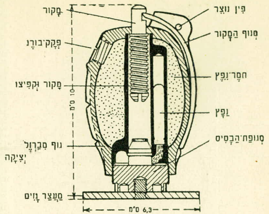
רימון "מילס" עם מעצור-זוים
