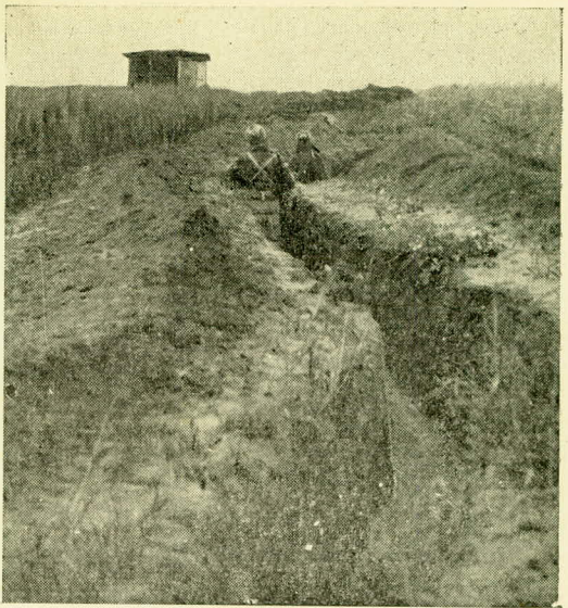
תעלת-קשר לעמדה חיצונית באחד הישובים העבריים
