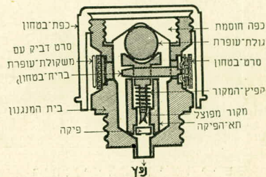
מנגנון-ההפעלה של רימונים בריטיים מס' 69 ו-73 (פרטים בטבלה שבעמוד 61)
