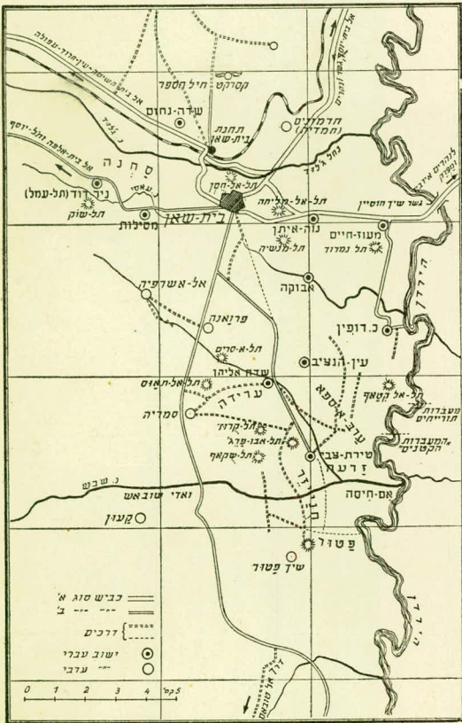
סביבת טירת-צבי ב-1948
