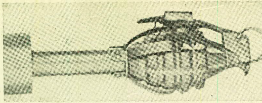
רימון יד שחורכב אליו מתקן המאפשר להטילו ע"י רובה.
