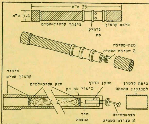
מרחם סכמטי של להביוור-היד הגרמני החדש
