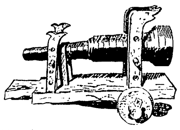
שלב נוסף: כנו של תותח-מצור זה (סוף המאה הייט) מאפשר כבר הגבהה או הנמכה מסוימת.
