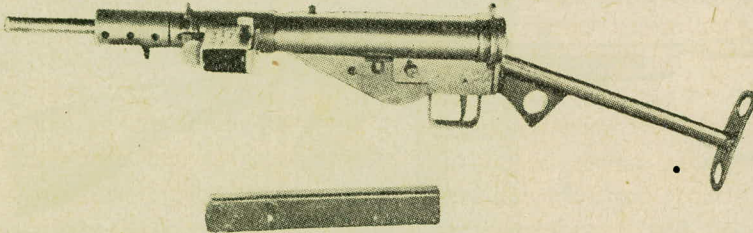
תת-מקלע „סטן” סימן II, קוטר 9 מ"מ; למטה: מחסנית מלבנית ומכילה 32 כדור
