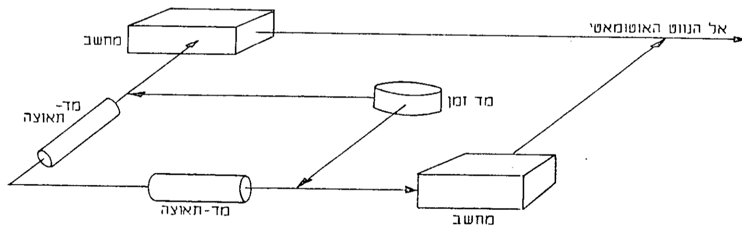
מערכת הנחיה אינרטיית
