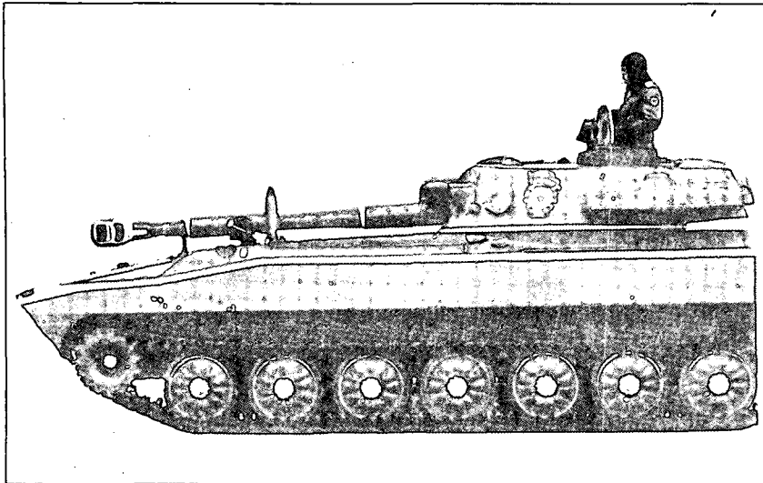
תומ"ת חדיש 122 מ"מ מדגם M-1974
