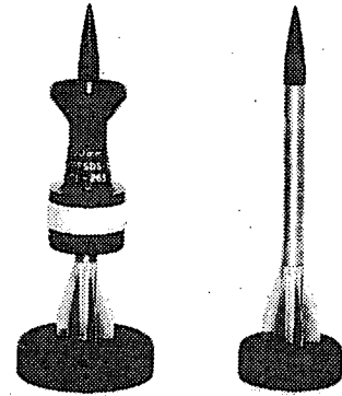
פגזי 60 מ"מ — מימין לשמאל: קליע, חדרון ופגז ח"ש מנעל מירוצב-סנפירים ופגז נפץ
