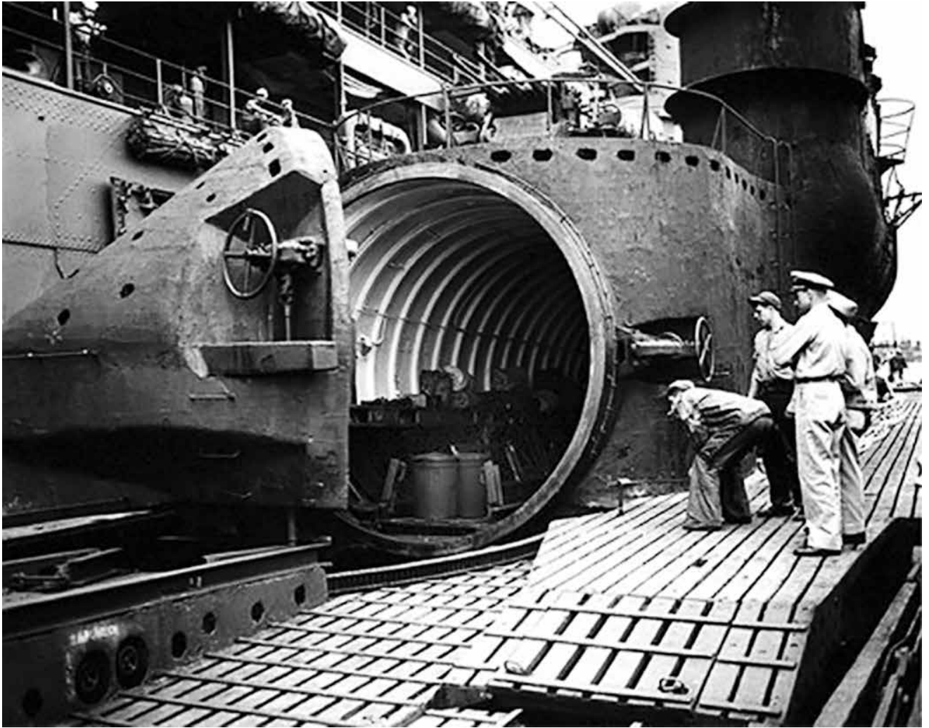
צוללת נושאת מטוסים יפנית מדגם I400. צוללות בודדות ביצעו מעללים כמו הפגזת קליפורניה או הפצצת יערות באורגון באמצעות מטוס המשוגר מהצוללת, עניין חדשני ובלתי מועיל למדי. צילום: ויקיפדיה
