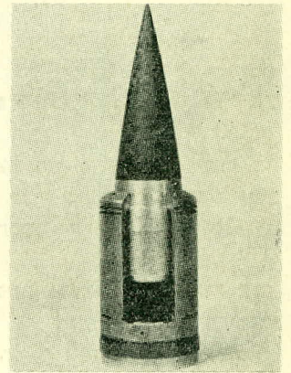
פגז חודר-שריון מנוע כשמנועו חתוך
