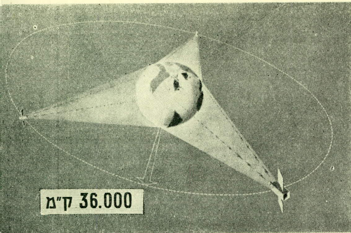
ציור מס' 4. תיאור סכמטי של עקרון פעולתו של לויין סינכרוני — ה"Advent". כל אחד משלושת הלויינים הסטציונריים משקיף על כשליש מכדור הארץ.
