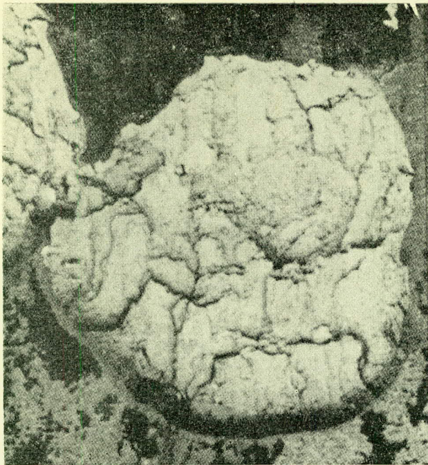
דופן פנימי של לוח שריון לאחר שנפגע ע"י פגז בעל ראש מעיך
