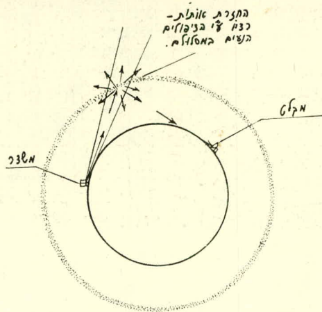
ציור מס' 5. תיאור טכני של תכנית "Dicon". מוצג כאן אופן פעולתה של הגורת המחטים הדו-קוטביים המשמשת כמחזיר גלי-רדיו בתחום הגלים האולטרה-קצרים
