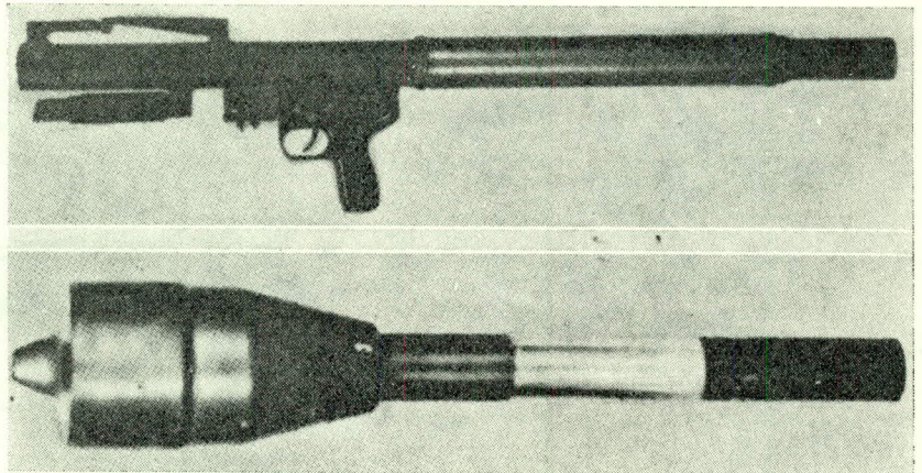
ה"פנצרובקה" (למעלה) והפצצה שלו (למטה)
