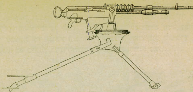
מכ"י הוצ'קים 1914, צרפתית. קוטר של 8 מ"מ, קירור אוויר. בשימוש צבא טוריה והלבנון
