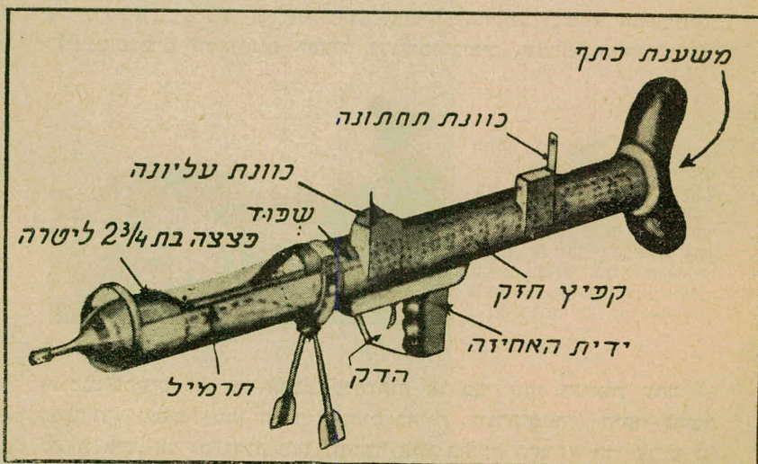
ה„פיאט“ (P.I.A.T.) — מטיל־פצצות אנטי־טנקי של חיל־הרגלים הבריטי. בשעת דחק עשוי להפעילו גם איש יחיד. טוח הפעולה האפקטיבי עד 115 יארד. מופעל גם נגד תיבות־שדה ובצורי־בטון. מצוי אצל ה„לגיון“ וחיל־הספר לעבה“.
