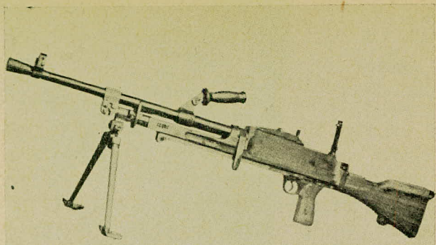
מקלע „ברן“ הנהוג בצבא הבריטי; קוטר 0.303; קירור אוויר; ניתן לשמש כזינוק וכמקלע־רגלים. מקובל בצבאות עיראק, עבה״י, מצרים וכן בחיל־הספר לעבה״י; יתכן כי מצוי גם בחילות ערב־הסעודית ובטוריה
