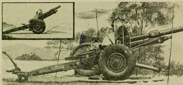
„תותח־הוביצר“ פגזו בן 25 ליטראות. כעת — הכלי העיקרי בארטי לרית השדה הבריטית. בצילום הקטן הוא מוצג במצב־יריה נוסח הוביצר — דהיינו, תוך הגבהת קנה־היריה, כדי שמסלול תעופת הפגז יהיה תלול יותר. טוח אשו היעילה כמות, עולה על 10 ק”מ.
