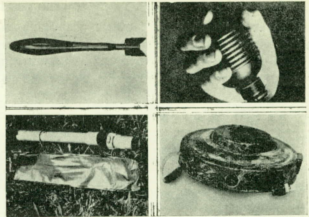
כלי-נשק נ"ט גרמניים: רימון-יד; אגרוף-שריון; מוקש נגד רכב; להביוור לשימוש חד-פעמי
