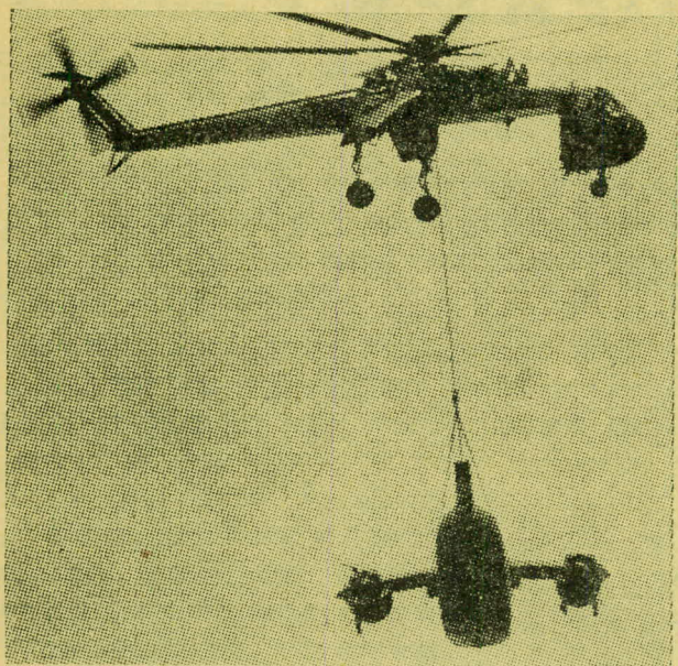
„העגרון המסופף“ מוביל מטוק „צ'ינוק“ שניזוק
