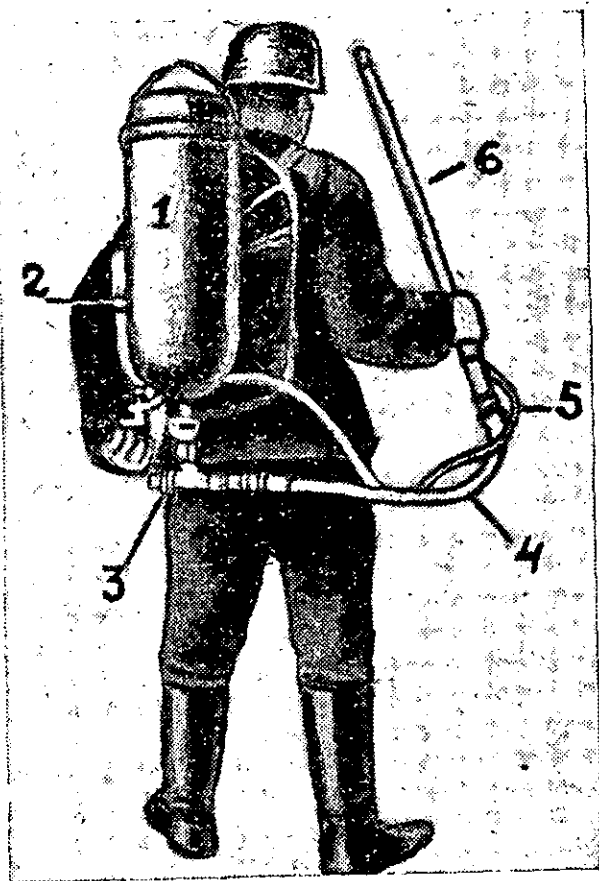
דוגמא של זרקאש גרמני 1. מיכל הדלק. 2. המיכל הקטן למימן דחום. לשם הצתת הדלק. 3. מפחת-לחץ. 4. צינור גמיש. 5. שסתום אבטומטי. 6. מסלנת.
