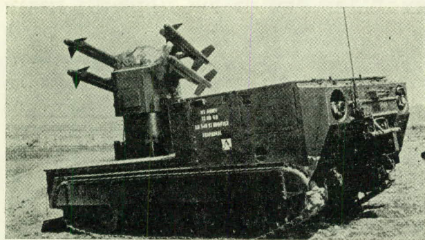
ננמ"ש נ"מ, צ'פארל", חמוש ב-4 טילים נ"מ מדגם "טיידוונדר"
