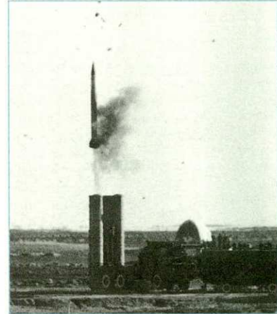
שיגור SA-10 בניסוי
