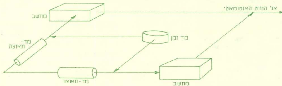
מערכת הנחיה אינרטיית
