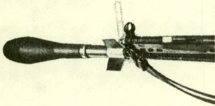
תמונה מס' 3: "G-3A4" עם רימון רובה; אין צורך בהתקן מיוחד ליריית הרימון.
