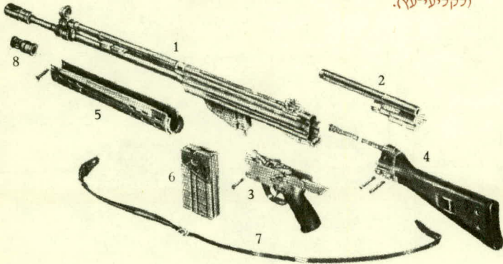
תמונה מס' 4: מכללי ה"ג-3": 1. הגוף עם הקנה, מערכת-הטעינה והכוונות; 2. המחלק; 3. בית-האחיזה עם מערכת-ההדק; 4. הקת; 5. המתפס; 6. המחסנית; 7. הרצועה; 8. מיצרי לוע (לקליע-עץ).
