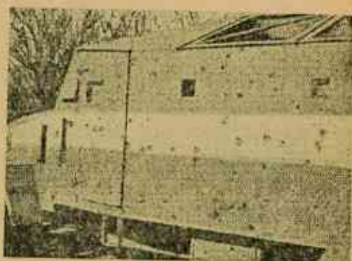
המשורין ש־ספג 250 קליעי כדורים
