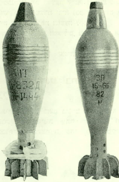
פצצה נפיצה ופצצת עשן למרגמה 82 מ"מ
