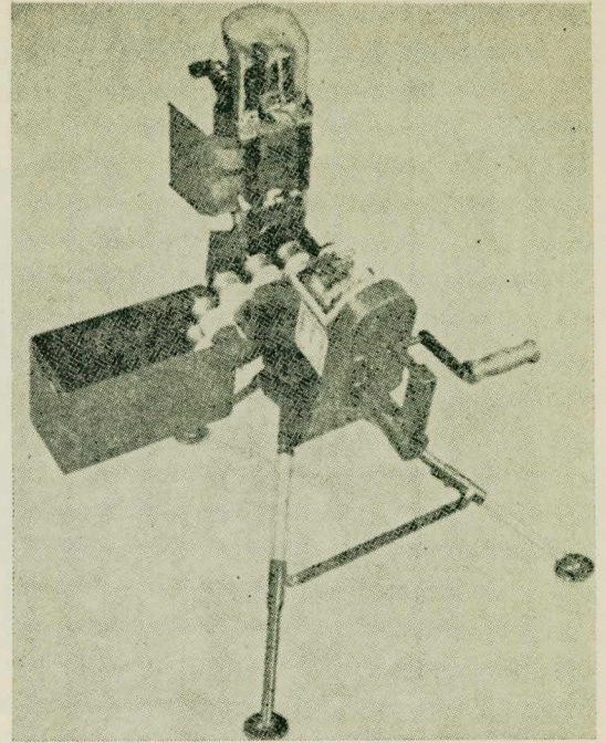
מקלע לתחמושת נפיצה 40 מ"מ
