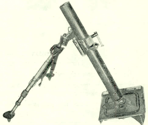
מרגמה 60 מ"מ „ברנט“
