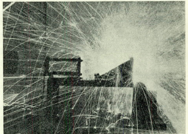
חץ אורניום בעת פגיעתו בלוח-שריון
