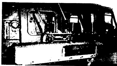
מיכל מוקשים להטלה ממטוק
