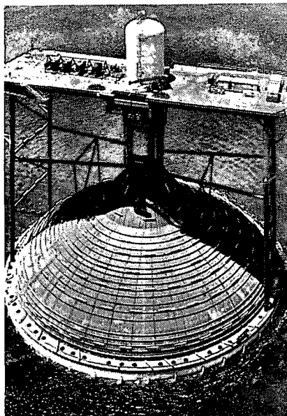
מכל תת קרקעי לאחסון נפט ליד חופי דובאי
