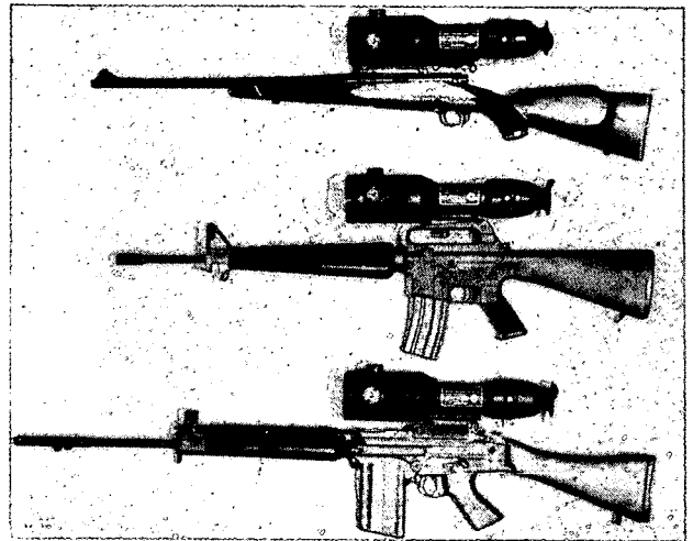
מגברי אור לרובים שונים, תוצרת Vero Inc's (ארצות-הברית).
