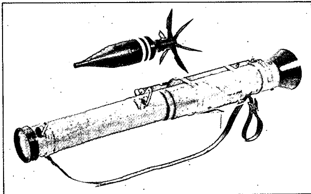
מטול (המועל לפי עקרון התול"ר) AT-4 (תוצרת שבדיה) האמור להחליף את ה-MINIMAN.
