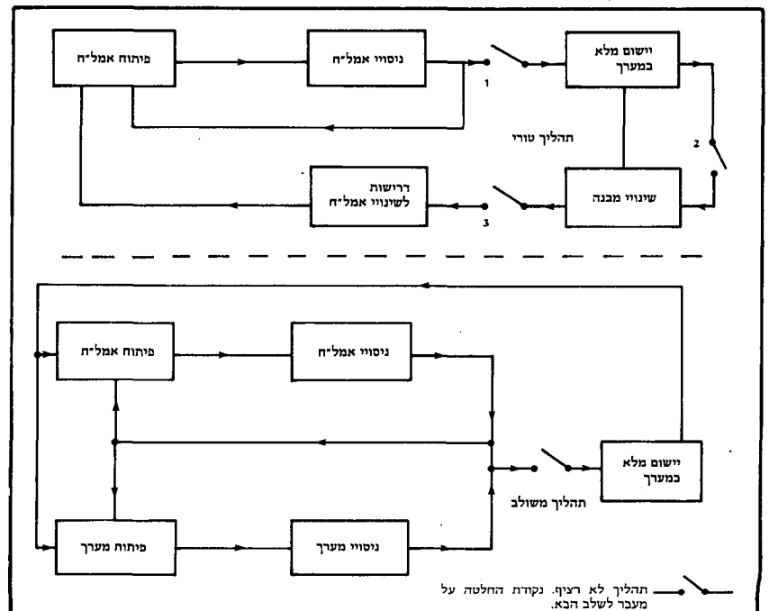
ציור מס' 3 השוואת תהליך טורי לתהליך משולב
